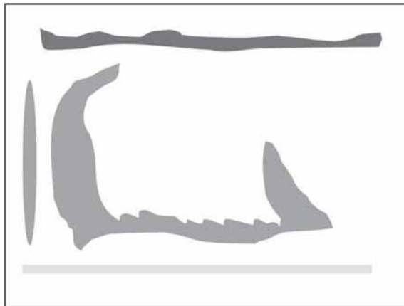
Fig. 8. Cromatograma de papel correspondiente a la separación de \beta -caroteno usando como fase móvil éter de petróleo
